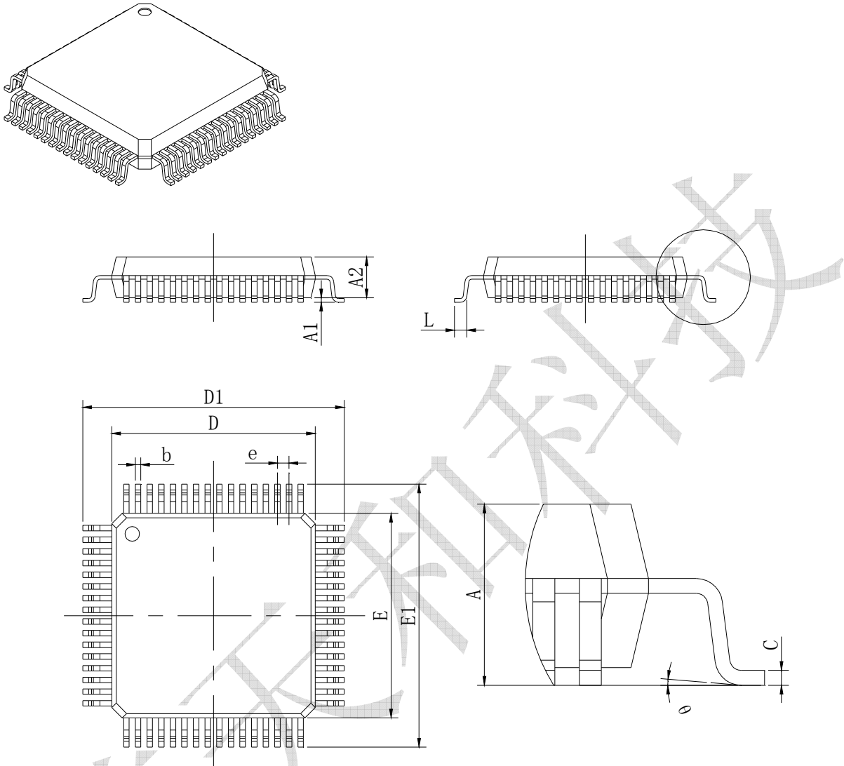
封装示意图 (LQFP64 7mm*7mm)
