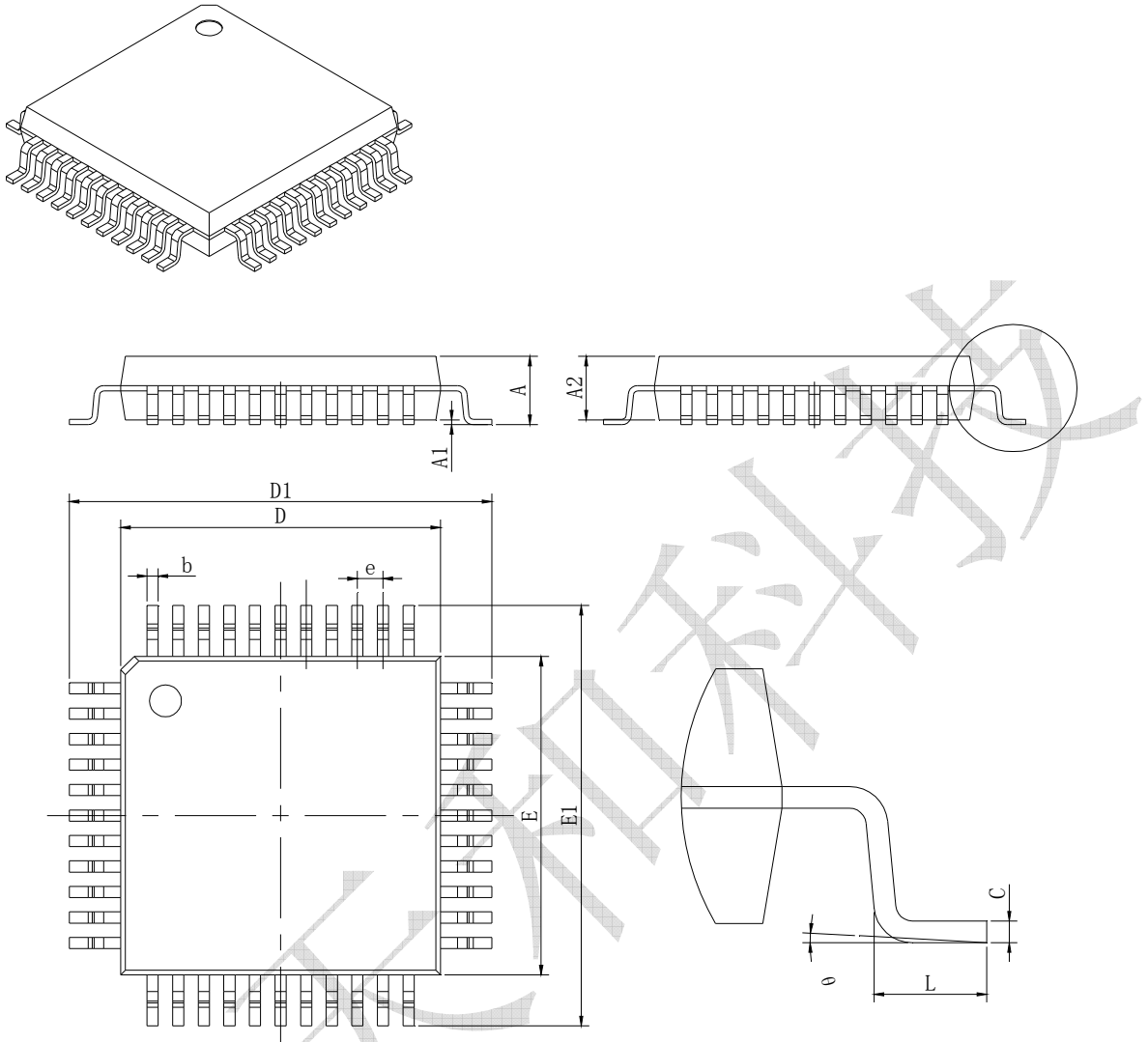
封装示意图 (LQFP44 10mm*10mm)
