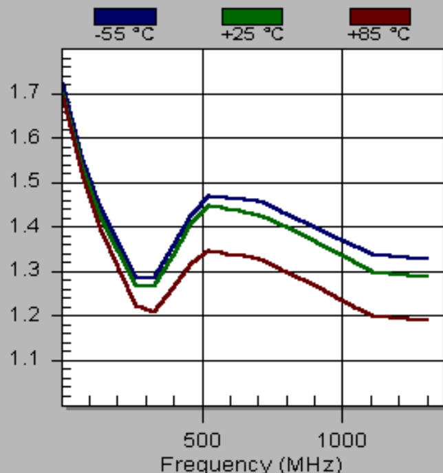
TM6212 Output VSWR
