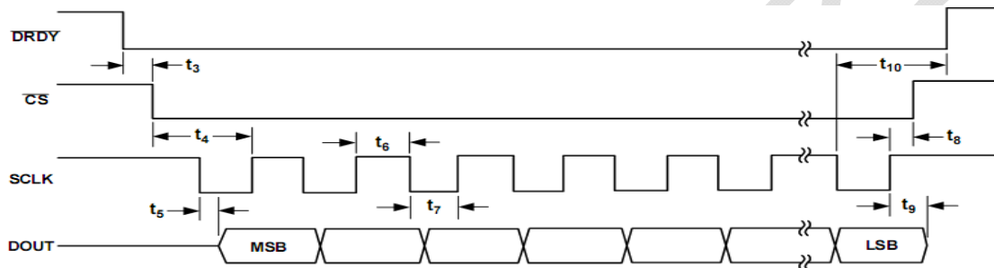
图 16 读周期时序图
