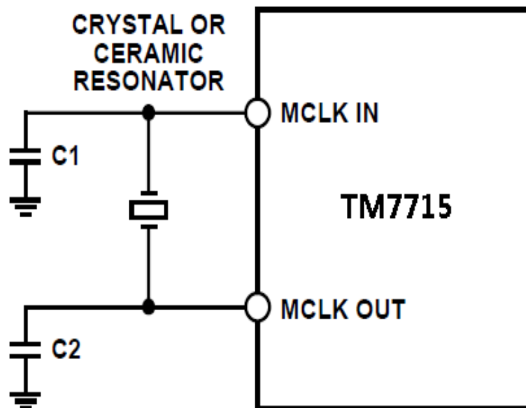
图 14 晶体或陶瓷谐振器与 TM7715 的连接
