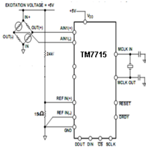
图 22 用 TM7715 作压力测量
