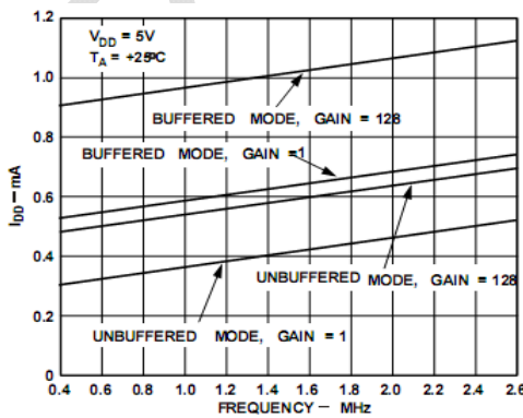
图6 I_{DD} 与MCLKIN 频率的关系 (5V电源电压)
