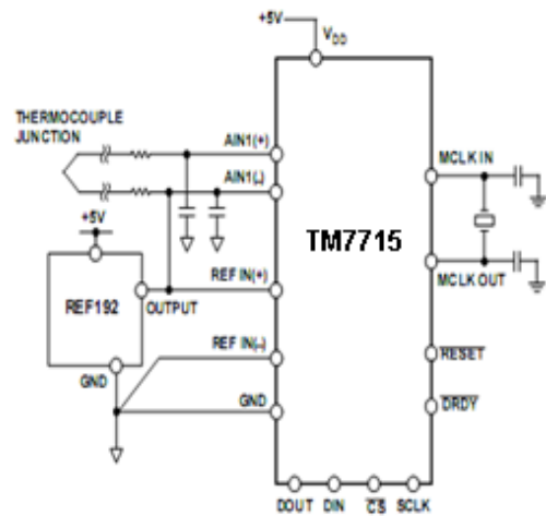
图 23 用 TM7715 作温度测量
