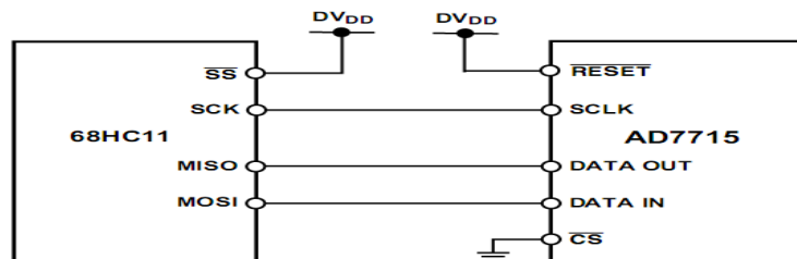
图 19 TM7715 与 68HC11
