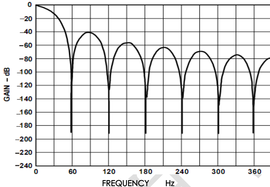
图 12 TM7715 滤波器的频率响应
