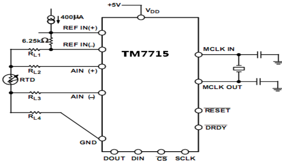
图 24 利用 TM7715 进行 RTD 测量
