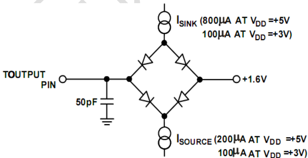
图1 访问时间和总线撤回时间的负载电路图
