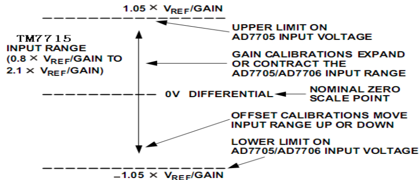
图13 输入范围和偏移的限制
