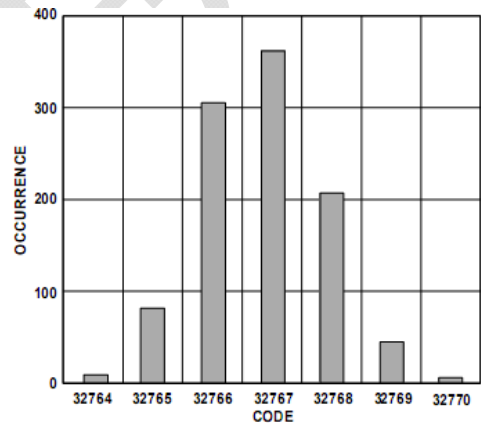
图5 图2中的数据分布图
