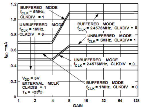
图7 I_{DD} 与增益和时钟频率的关系 (5V电源电压)
