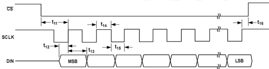
图 17 写周期时序图
