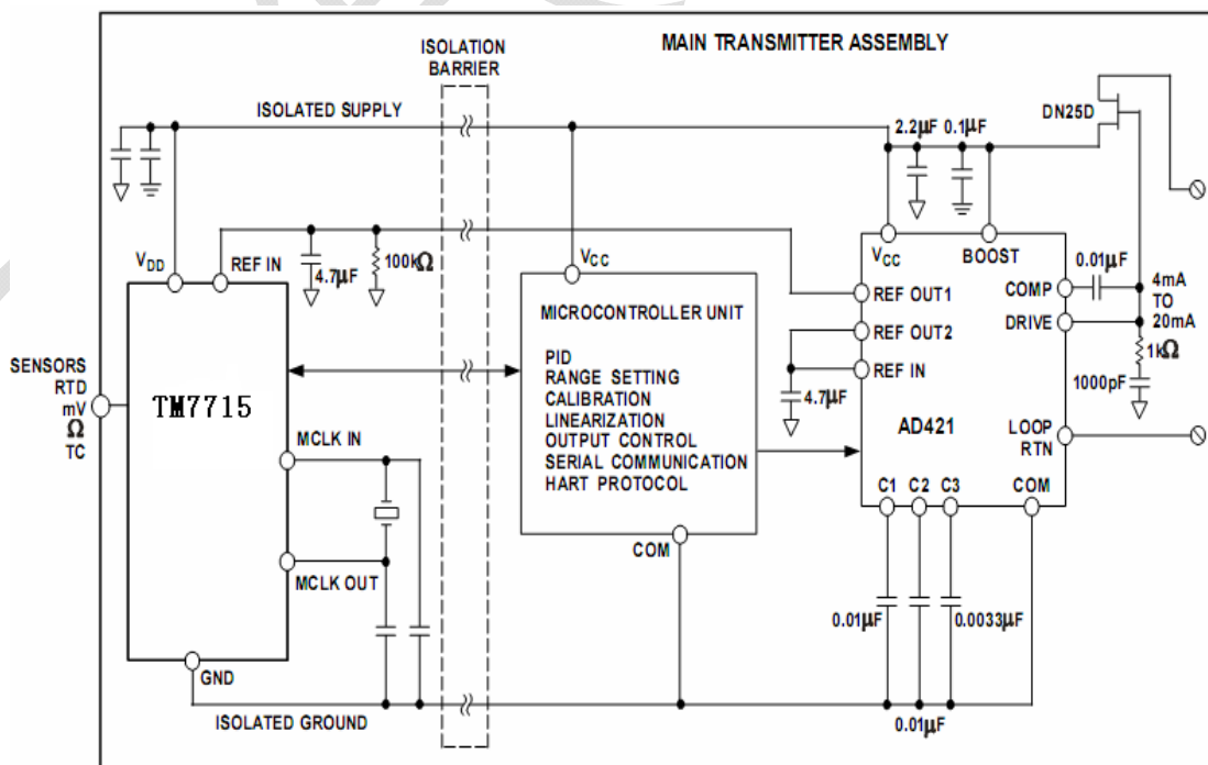
图 25 使用 TM7715 的智能发射器
