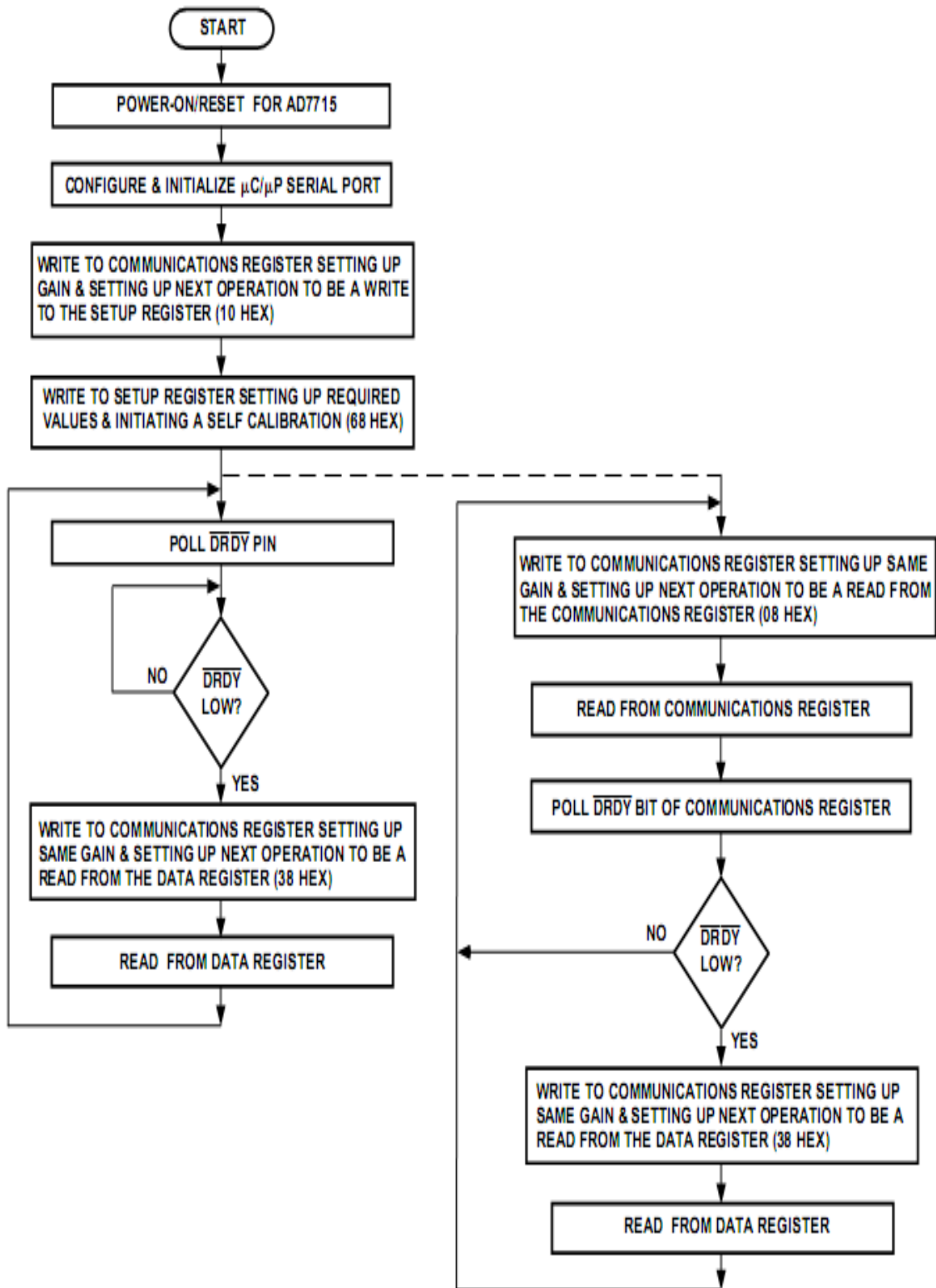
图 18 TM7715 的寄存器设置和读数流程图
