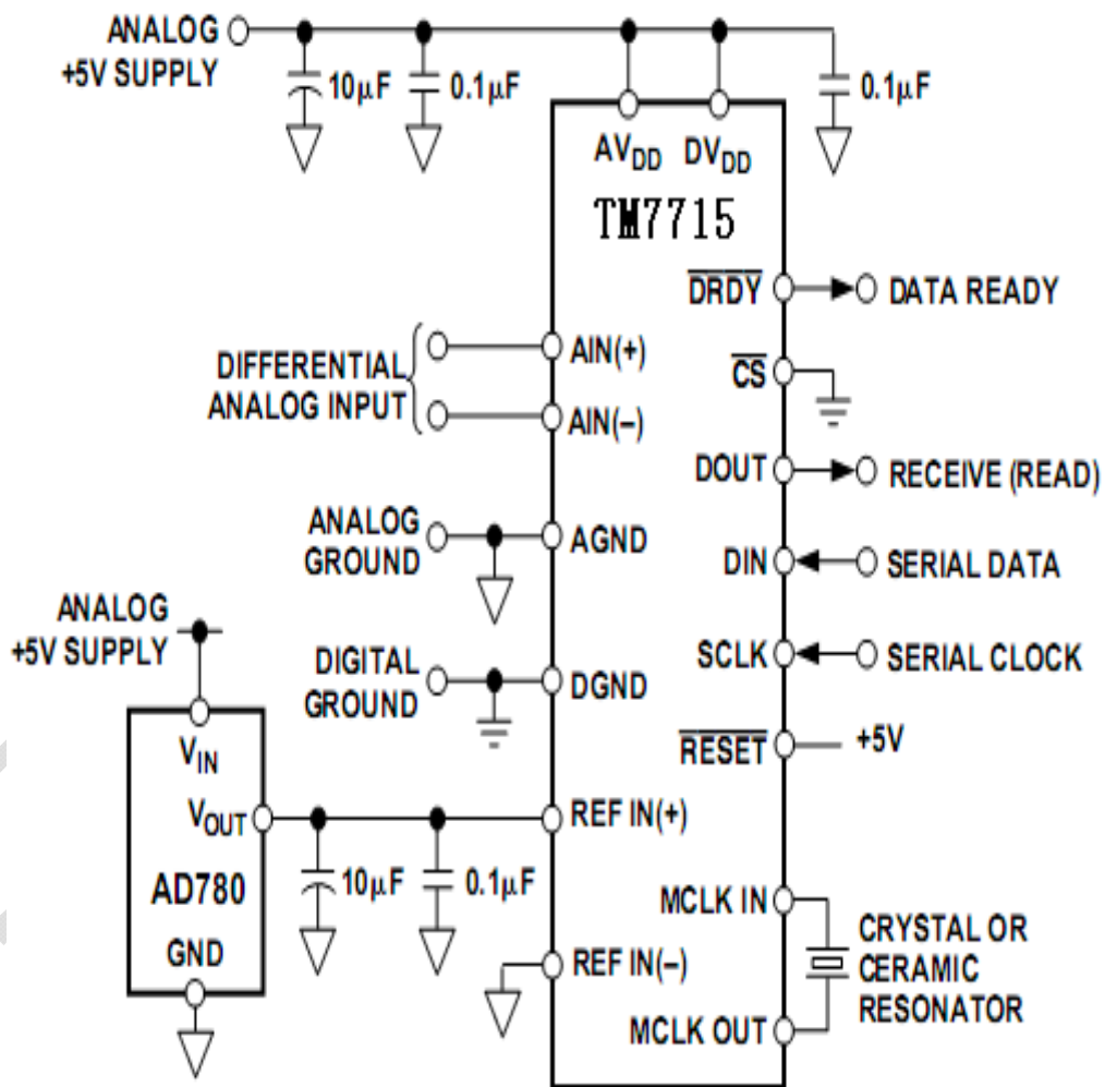
图 10 TM7715 的基本连接电路图
