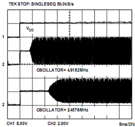
图8 典型晶体振荡器上电时间
