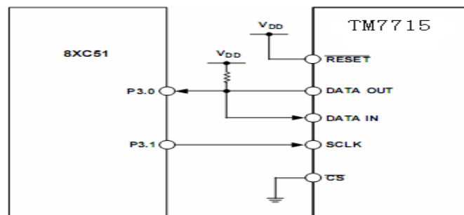
图 20 TM7715 与 8x51 接口
