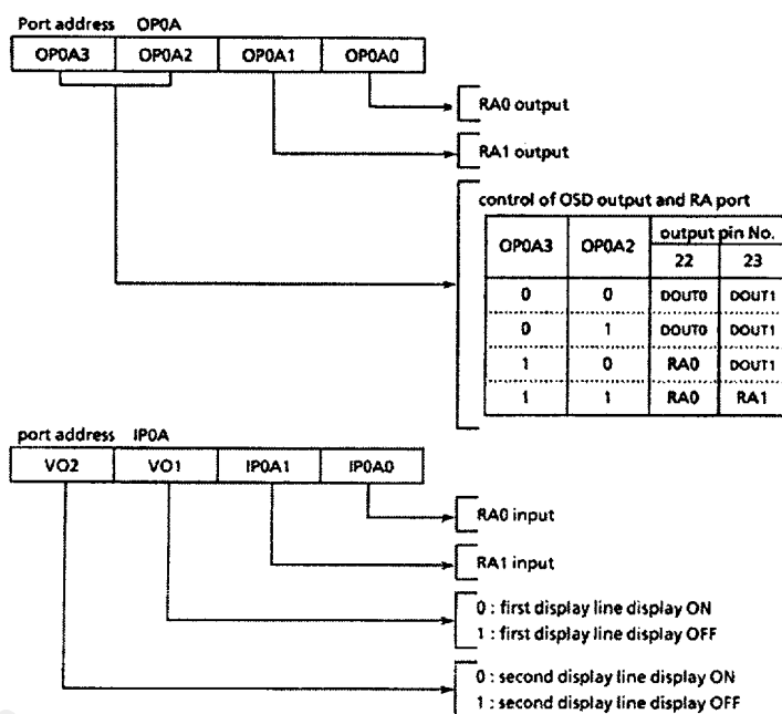
Figure 3-9. Port RA
