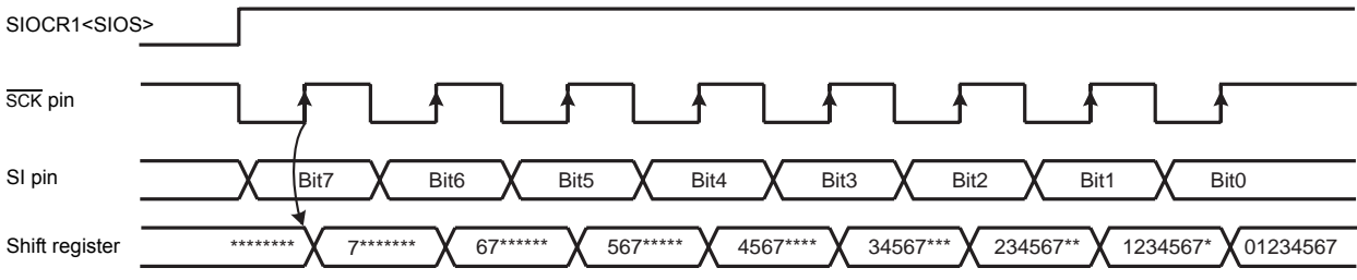
Figure 9-4 Shift Edge
