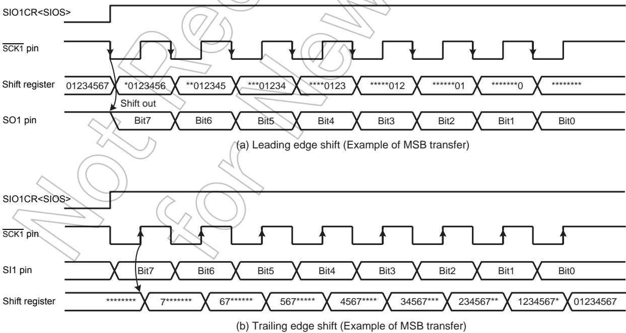
Figure 14-4 Shift Edge
