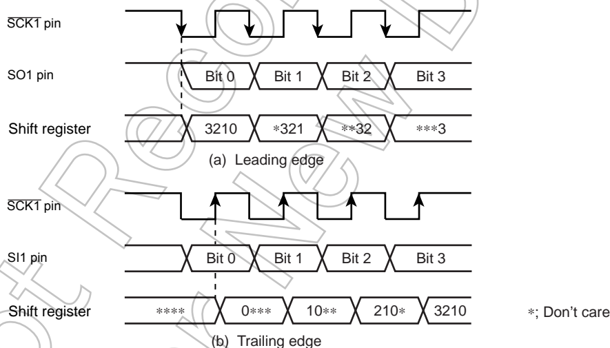
Figure 15-5 Shift edge
