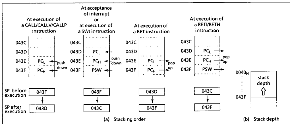
Figure 1-8. Stack
