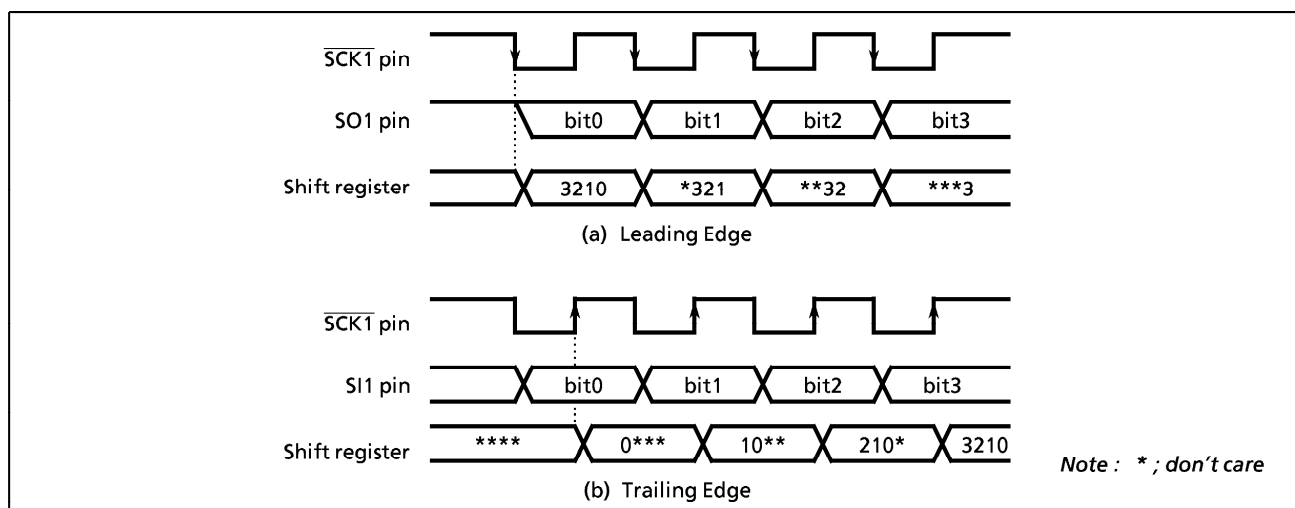
Figure 2-52. Shift Edge
