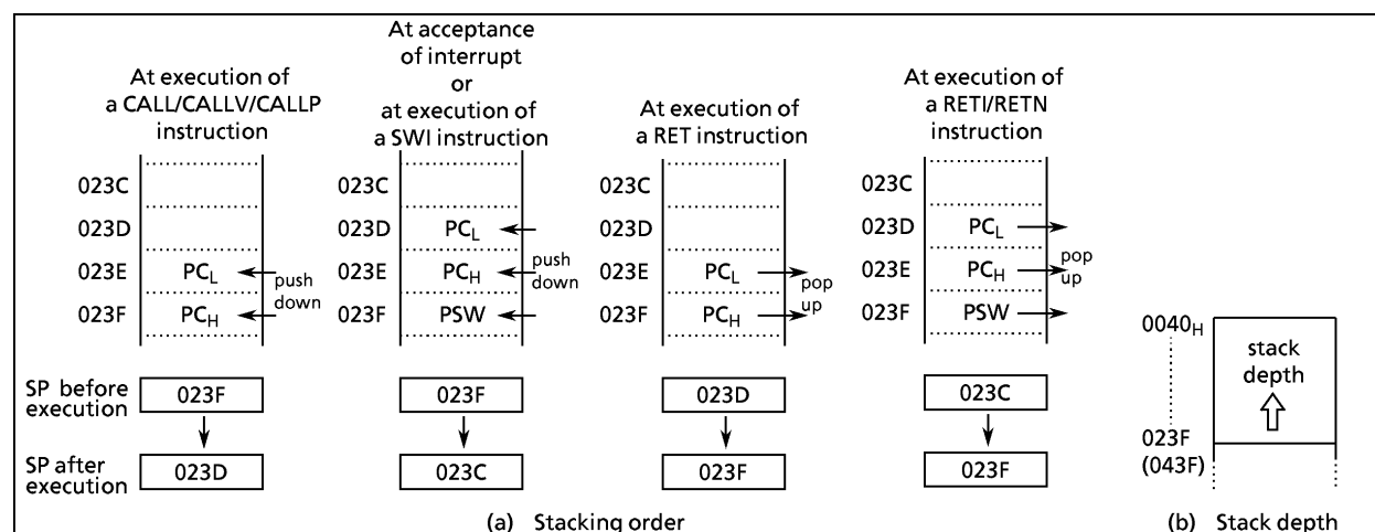
Figure 1-8. Stack
