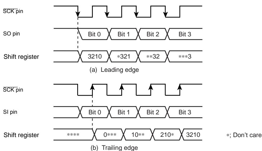
Figure 16-5 Shift edge
