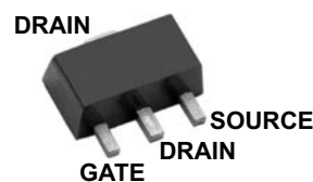
TO-243AA (SOT-89) (N8)
