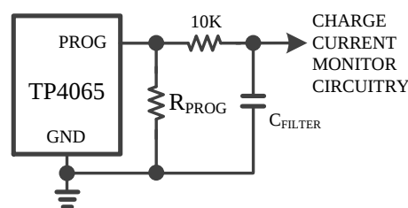
图5：隔离 PROG 引脚上的容性负载和滤波电路
