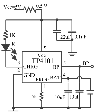
TP4101 单灯 0.6A 充电电池管理电路
