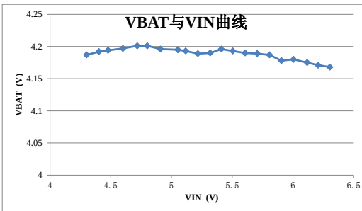
截止电压与电源电压关系
