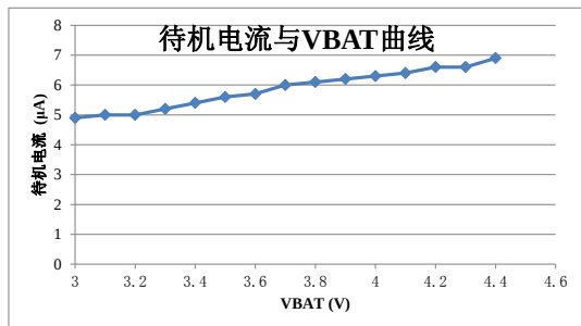
待机电流与电池电压的关系
