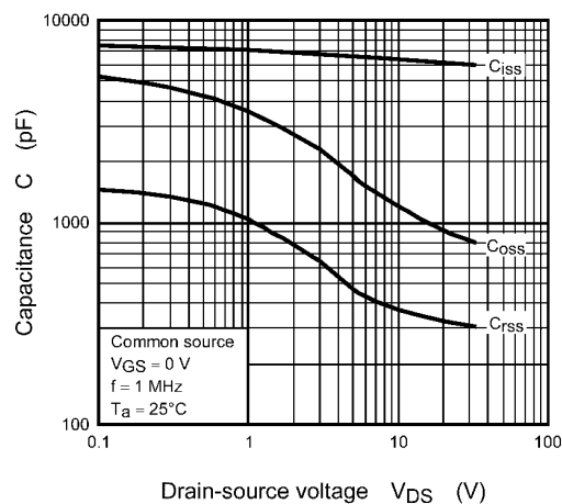
Fig. 8.8 Capacitance - V_{DS}
