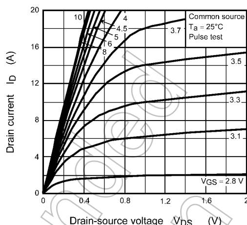
Fig. 8.2 I_D - V_{DS}
