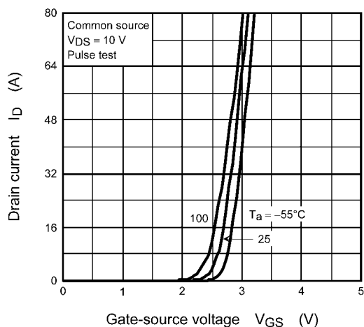
Fig. 8.3 I_D - V_{GS}
