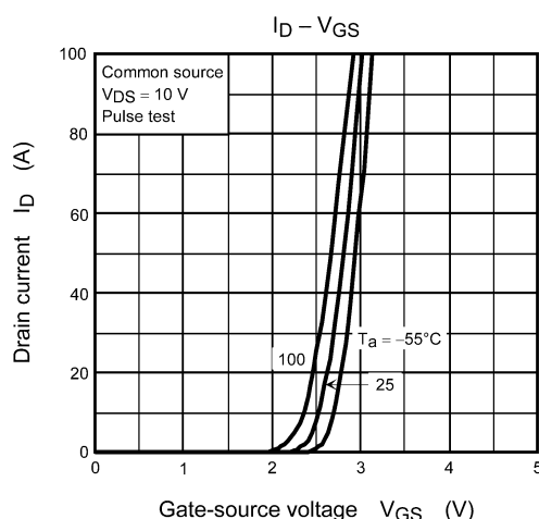
Fig. 8.3 I_D - V_{GS}
