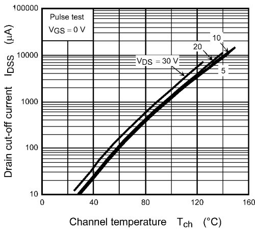
Fig. 8.16 I_{DSS} - T_{ch}
