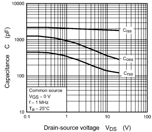
Fig. 8.8 Capacitance - V_{DS}
