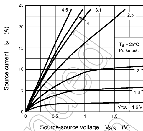
Fig. 10.2 I_S - V_{SS} (Note 6)
