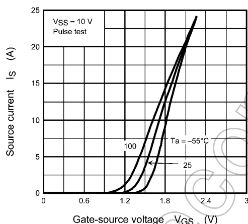
Fig. 10.3 I_S - V_{GS} (Note 5)
