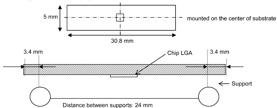
Fig. 9.4.1 Placement
