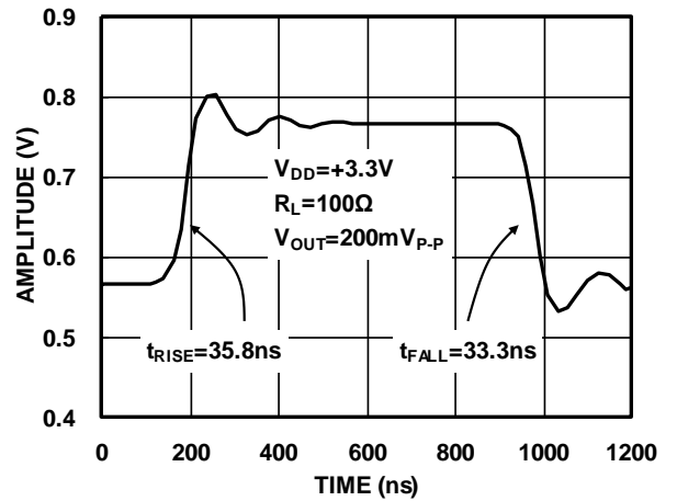
图10. 小信号脉冲响应特性 (SD Channel)
