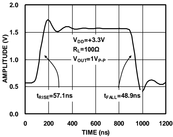
图9. 大信号阶跃响应瞬态特性 (SD Channel)
