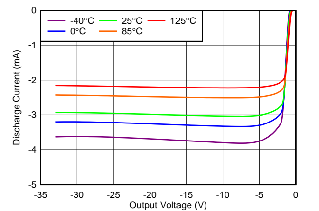
Figure 53. I_{NR/SS} vs V_{NR/SS}
