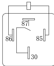
1A 接线图
