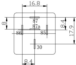
安装图 (快连接式)
