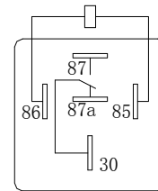
1C 接线图
