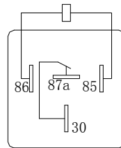
1B 接线图
