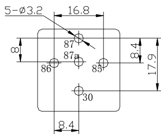
安装图(PCB)
