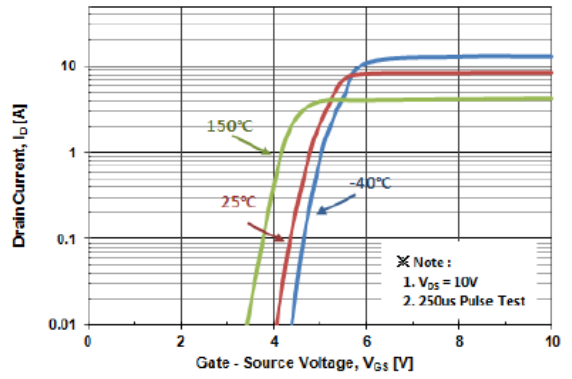
Fig. 2 I_D - V_{GS}
