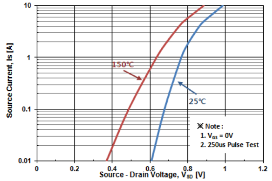
Fig. 4 I_S - V_{SD}
