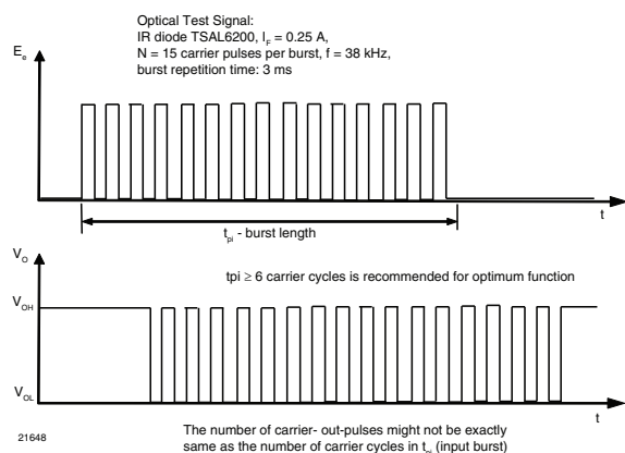
Fig. 1 - Output Function
