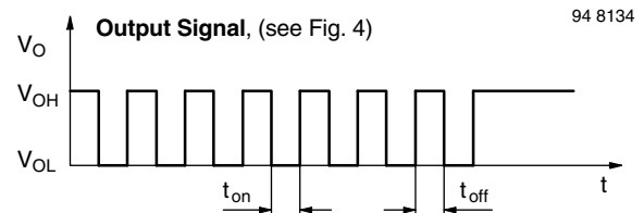
Fig. 3 - Output Function
