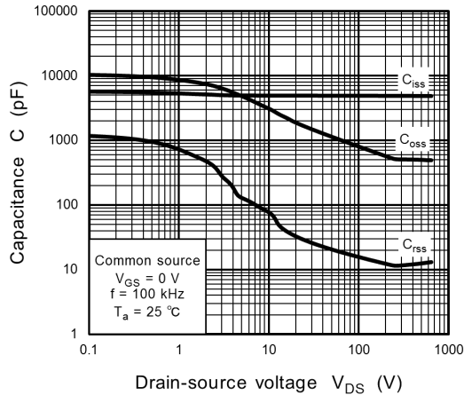
Fig. 8.13 C - V_{DS}
