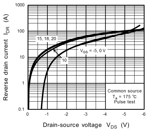
Fig. 8.10 I_{DR} - V_{DS}
