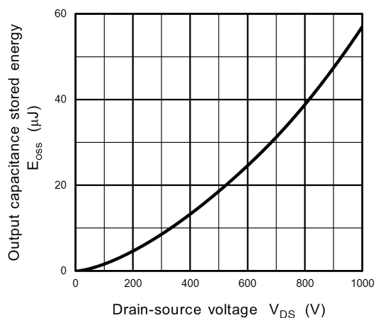
Fig. 8.14 E_{oss} - V_{DS}
