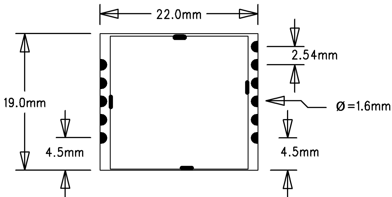
顶视图
