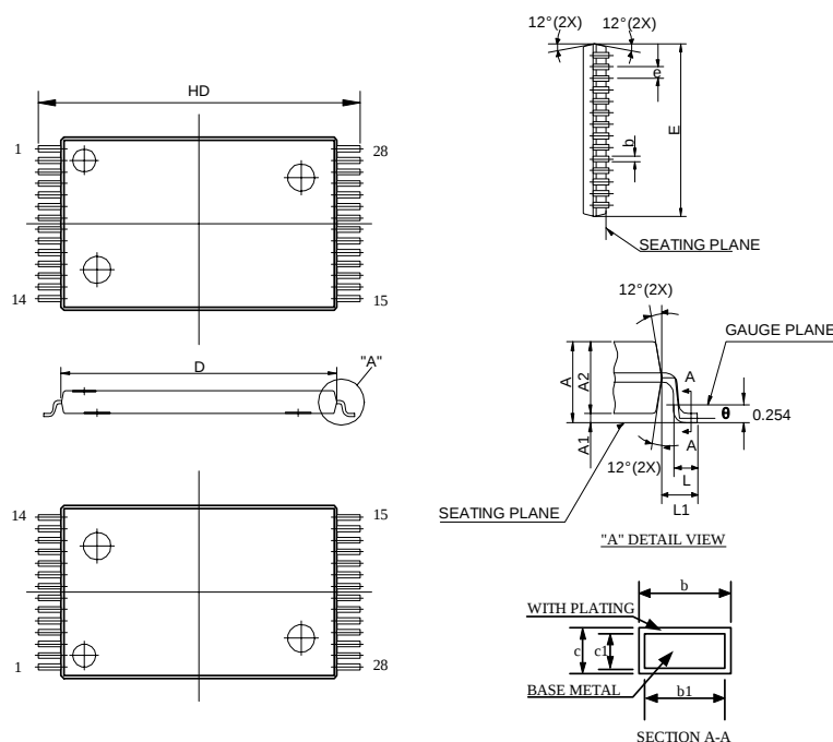
TSOP - 28
