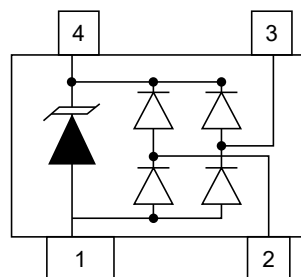
SOT-143
