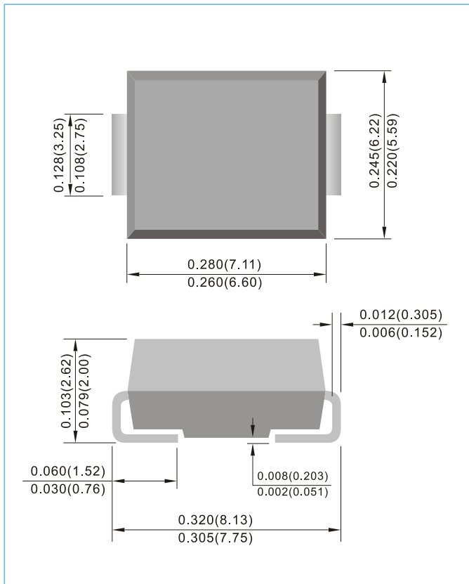
SMC / DO-214AB Unit : inch(mm)
