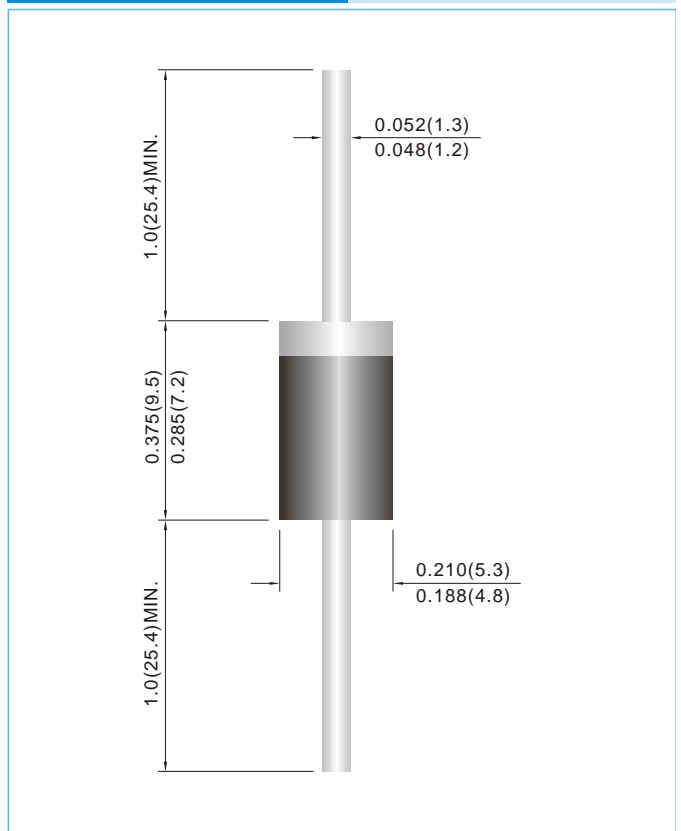
DO-201AD Unit : inch(mm)
