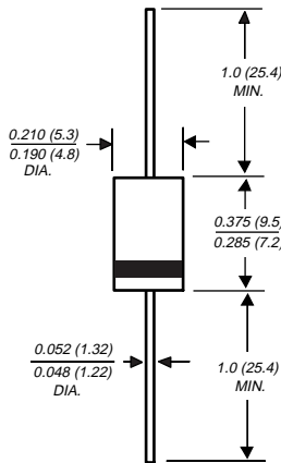
DO-201AD
