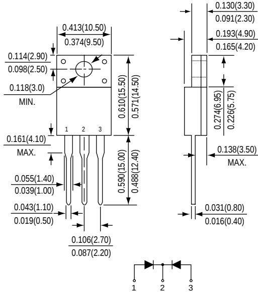
ITO-220AB
