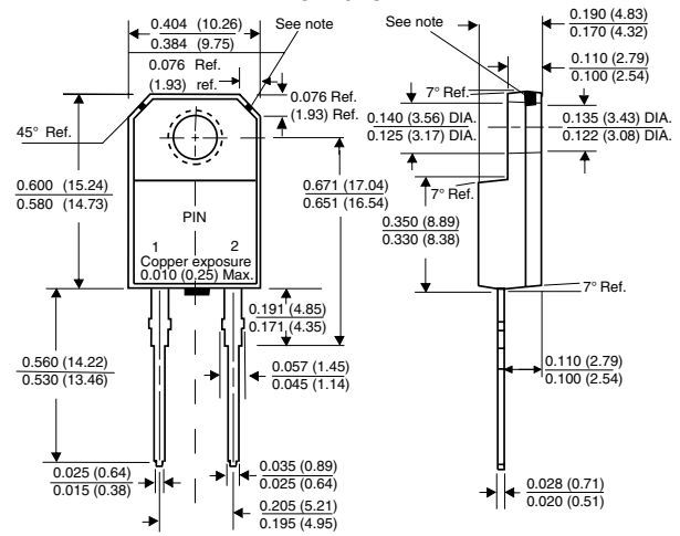
ITO-220AC
