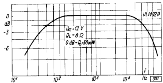
Wzmocnienie napięciowe w funkcji częstotliwości
