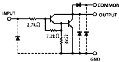
ULN2803AP/AFW
