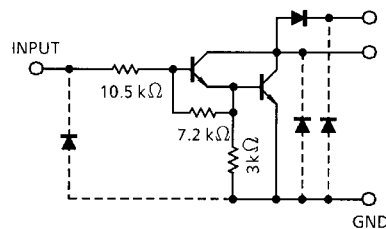
ULN2804AP / AFW
