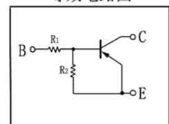
等效电路图
