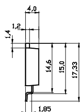
USS 4-T220 / UNS 4-T220
