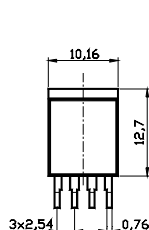
USS 4-T220 / UNS 4-T220
