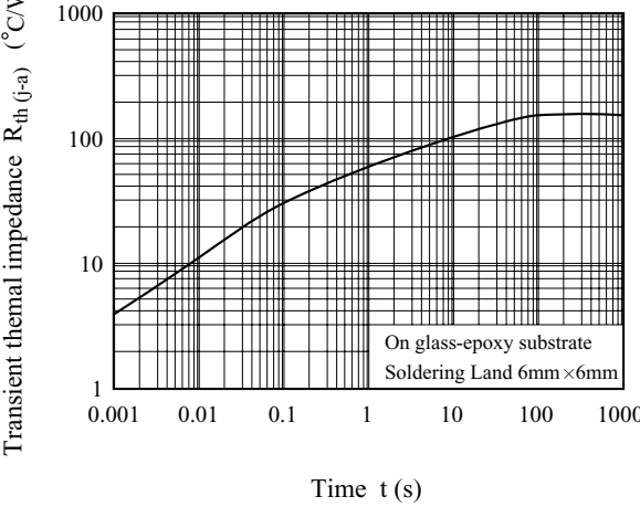
R_{th(j-a)} - t
