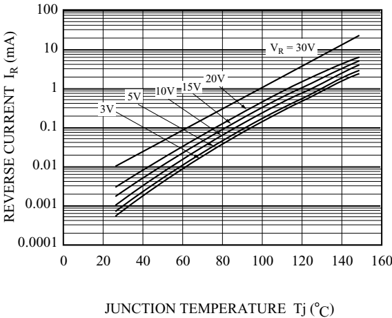
I_R - T_j
