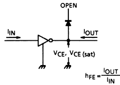
2. V_{CE(sat)} , h_{FE}
