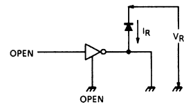
6. I_R
