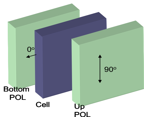
LCD module
