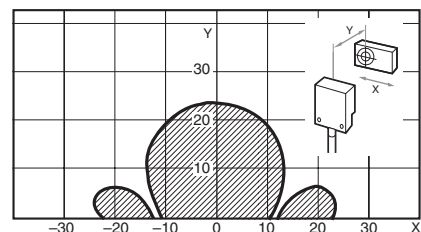
V600-HS61 & V600-D8KR12
