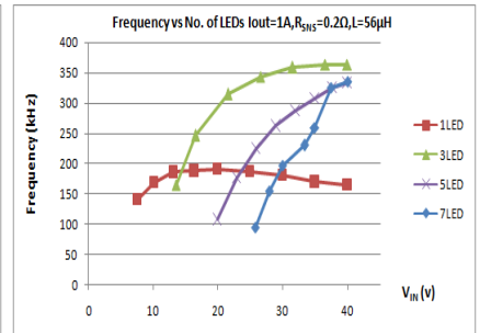
Vin vs. Frequency R_{SNS}=0.2\Omega, L=56\mu H
