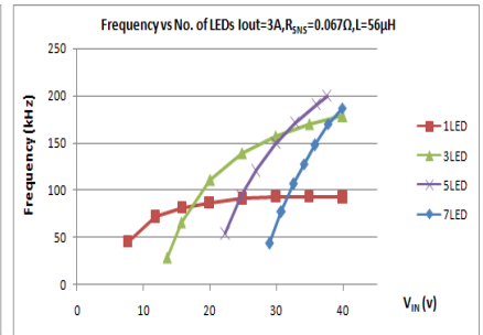
Vin vs. Frequency R_{SNS}=0.067\Omega, L=56\mu H
