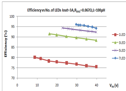
Vin vs. Efficiency R_{SNS}=0.067\Omega, L=100\mu H
