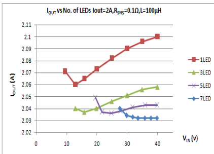
Vin vs. I_{OUT} R_{SNS}=0.1\Omega, L=100\mu H
