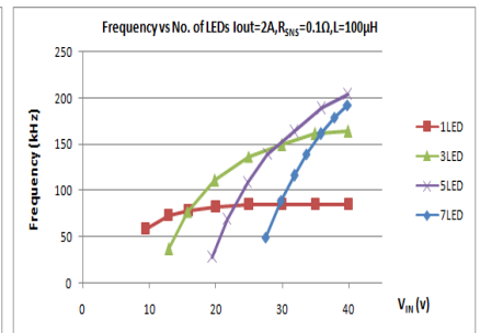
Vin vs. Frequency R_{SNS}=0.1\Omega, L=100\mu H
