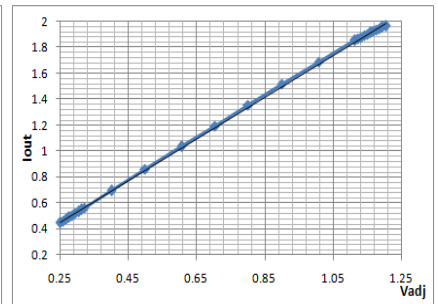
Vadj vs. IOUT R_{SNS}=0.1\Omega, L=100\mu H
