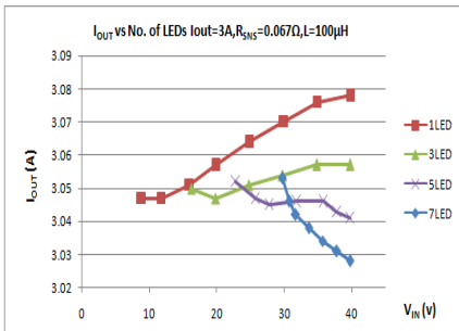
Vin vs. IOUT R_{SNS}=0.067\Omega, L=100\mu H
