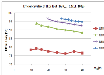
Vin vs. Efficiency R_{SNS}=0.1\Omega, L=100\mu H
