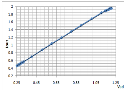
Vadj vs. IOUT R_{SNS}=0.1\Omega, L=56\mu H
