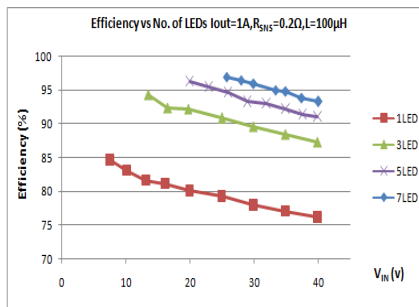
Vin vs. Efficiency R_{SNS}=0.2\Omega, L=100\mu H
