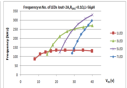
Vin vs. Frequency R_{SNS}=0.1\Omega, L=56\mu H
