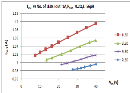
Vin vs. I_{OUT} R_{SNS}=0.2\Omega, L=56\mu H
