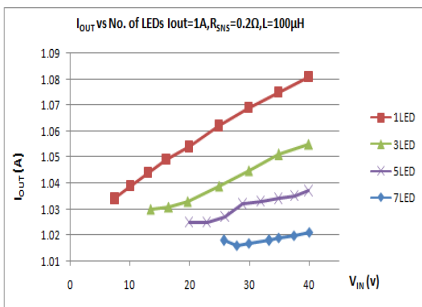
Vin vs. I_{OUT} R_{SNS}=0.2\Omega, L=100\mu H
