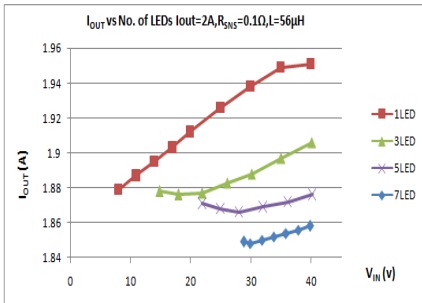
Vin vs. I_{OUT} R_{SNS}=0.1\Omega, L=56\mu H
