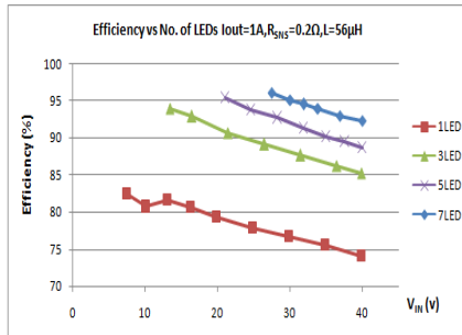
Vin vs. Efficiency R_{SNS}=0.2\Omega, L=56\mu H
