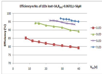
Vin vs. Efficiency R_{SNS}=0.067\Omega, L=56\mu H
