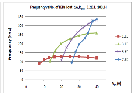
Vin vs. Frequency R_{SNS}=0.2\Omega, L=100\mu H
