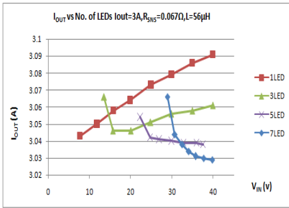
Vin vs. IOUT R_{SNS}=0.067\Omega, L=56\mu H
