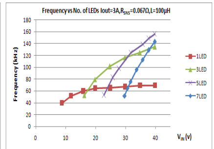
Vin vs. Frequency R_{SNS}=0.067\Omega, L=100\mu H
